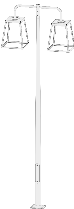
H 4 070 . L 452 . P 1390
